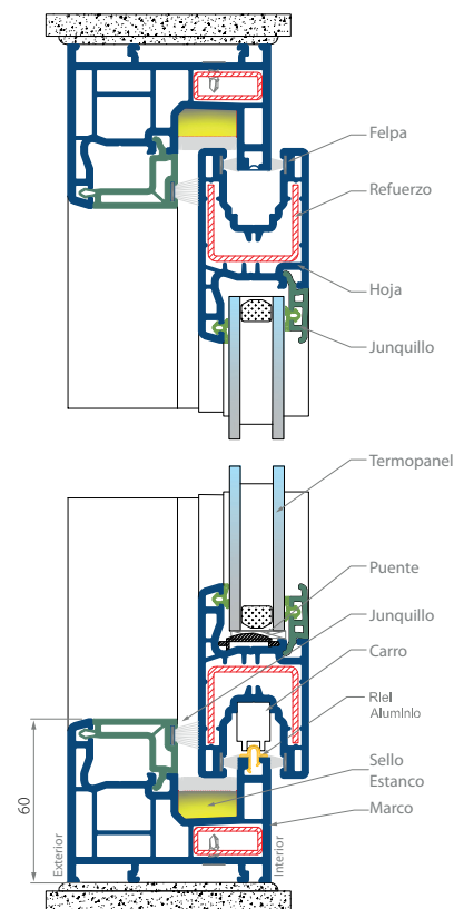
CORTE B-B
