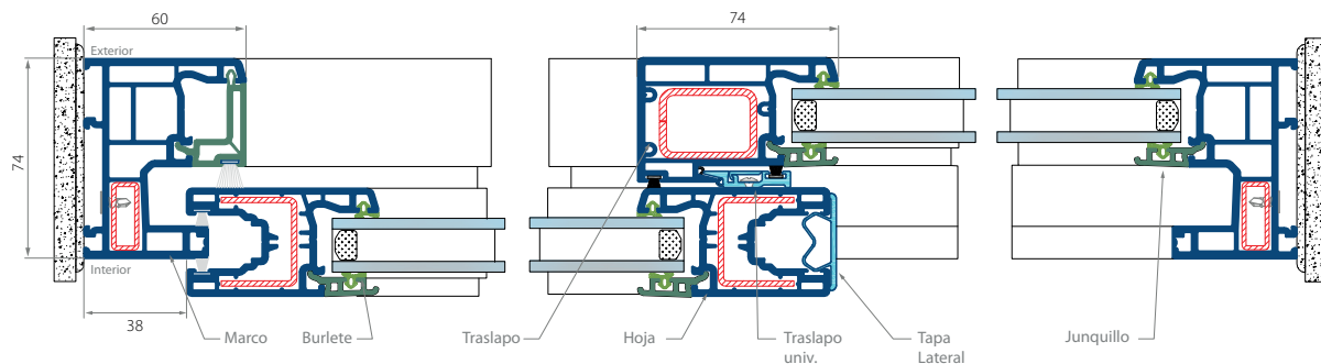
CORTE A-A
